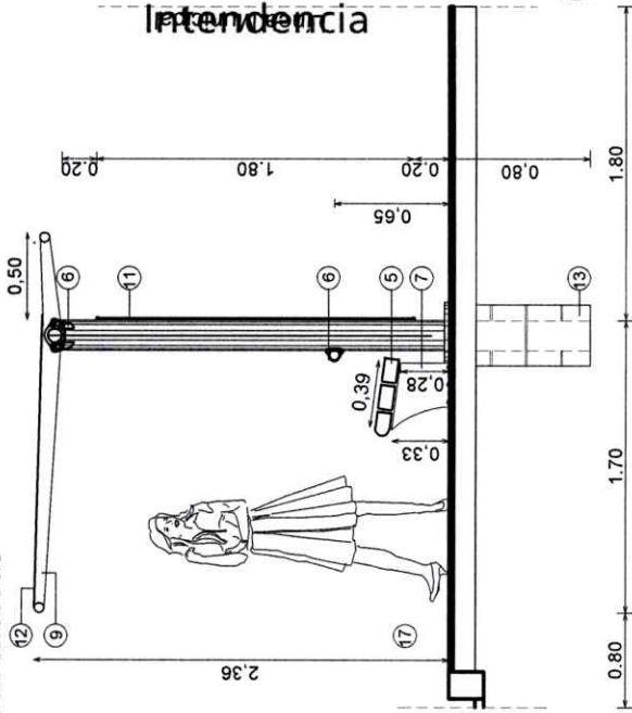
vista lateral
